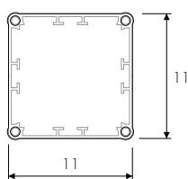
Pilier
